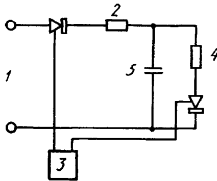
Тиристорная схема
