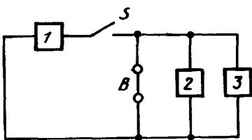
1 — источник постоянного напряжения; S — переключатель; B — переключатель; 2 — измеряемый конденсатор; 3 — запоминающий осциллограф
