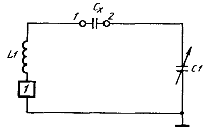
C_x — измеряемый конденсатор; CI — конденсатор переменной емкости; LI — индуктивная катушка связи; I — индикатор резонанса; 1, 2 — выводы схемы
